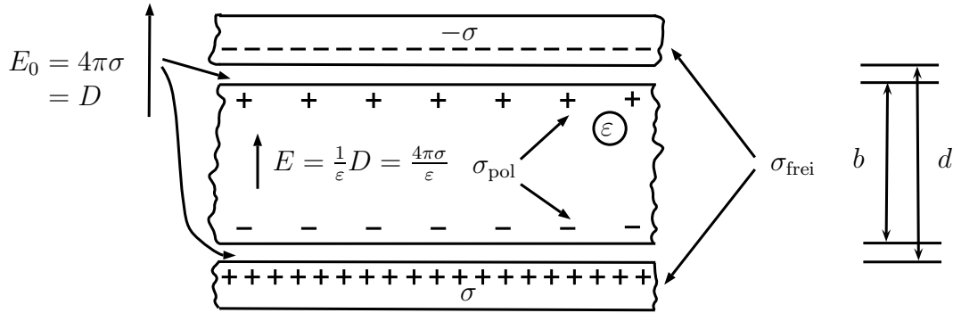
Abbildung 4.22: Plattenkondensator mit eingeschobenem Dielektrikum
