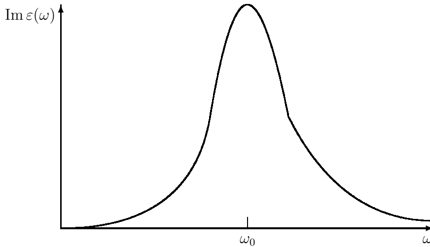
Abbildung 4.33: Schematischer Verlauf von \operatorname{Im} \varepsilon(\omega) im Oszillatormodel
