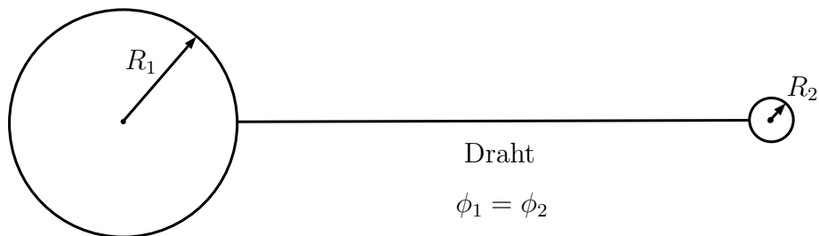
Abbildung 4.9: Zwei weit entfernte Metallkugel auf gleichem Potential
