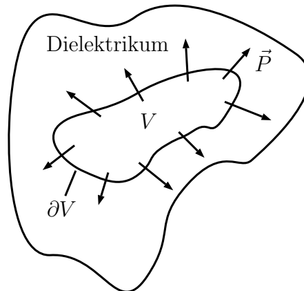
Abbildung 4.20: Räumlich inhomogene Dipoldichte in einem Dielektrikum
