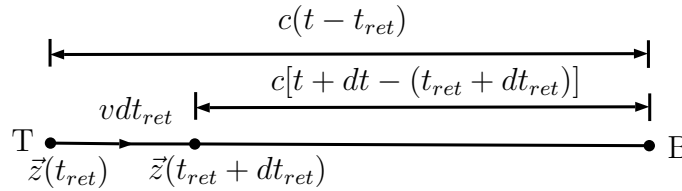
Abbildung 3.56: Zur Illustration des Zustandekommens des Unterschiedes zwischen dt_{\text{ret}} (Zeitintervall für das Teilchen T) und dt (Zeitintervall für den Beobachter B)
