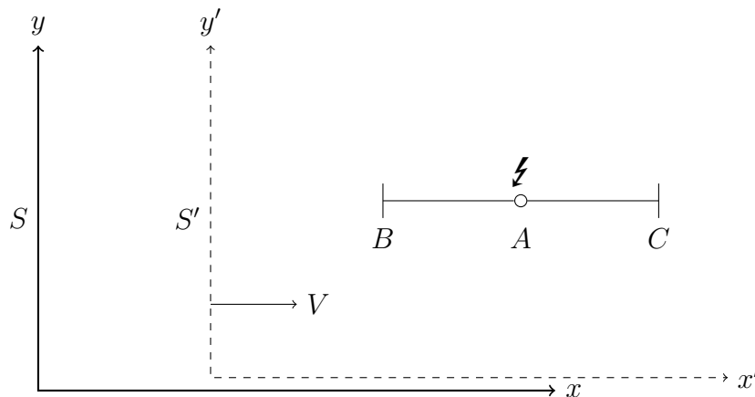
Abbildung 2.1: Inertialsystem S' bewegt sich mit Geschwindigkeit V relativ zu Inertialsystem S ; BAC ruht in S'
