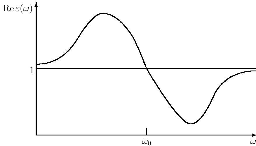
Abbildung 4.32: Schematischer Verlauf von \text{Re } \varepsilon(\omega) im Oszillatormodell
