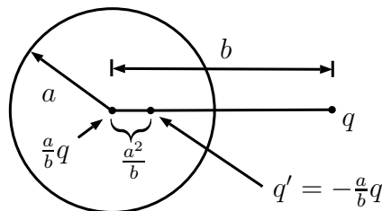
Abbildung 4.16: Isolierte leitende Kugel
