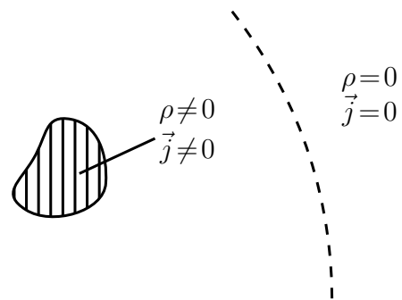
Abbildung 3.6: Ladungs- und Stromverteilung
