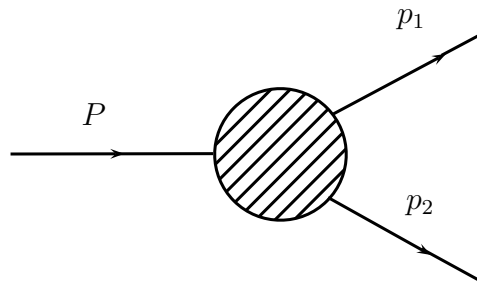
Abbildung 2.13: Zerfall eines Teilchens mit Viererimpuls P in zwei Teilchen mit Viererimpulsen p_1, p_2
