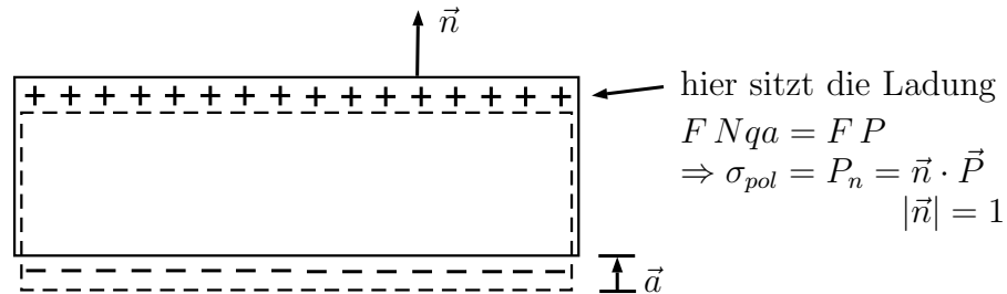
Abbildung 4.19: Dielektrikum bei angelegtem äußerem Feld
