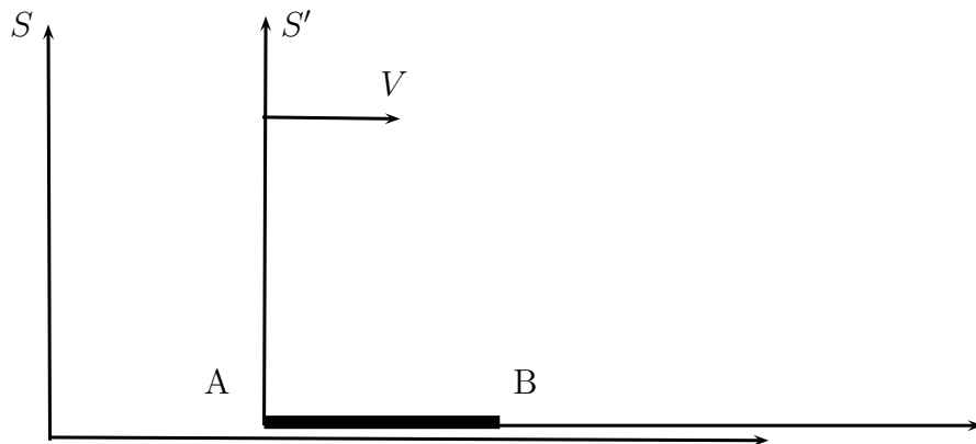
Abbildung 2.5: Stab AB ruht in S'
