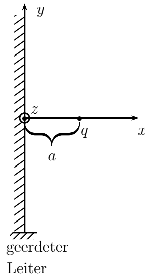
Abbildung 4.14: Geerdeter Leiter in der y - z -Ebene, im Abstand a die Punktladung q
