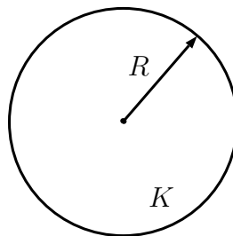
Abbildung 4.8: Geladene Kugel
