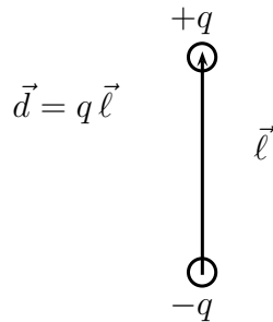
Abbildung 3.15: Prototyp eines elektrischen Dipols
