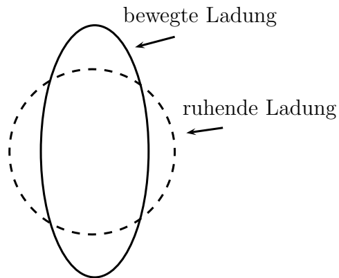
Abbildung 3.12: Flächen mit gleichem Betrag der Feldstärke
