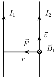
Abbildung 3.22: Kraft zwischen zwei stromdurchflossenen, unendlich langen, parallelen Drähten
