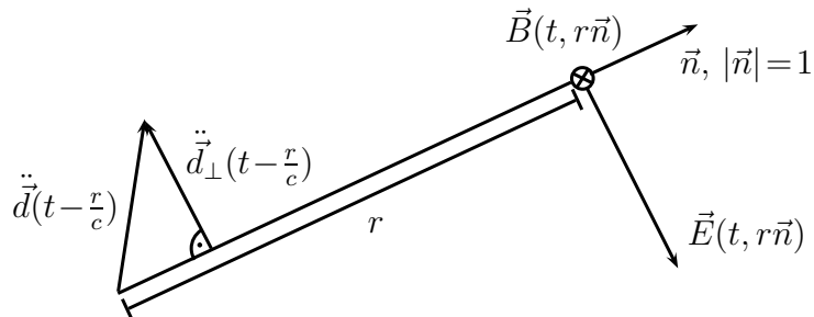
Abbildung 3.51: Strahlungsfeld in Dipolnäherung
