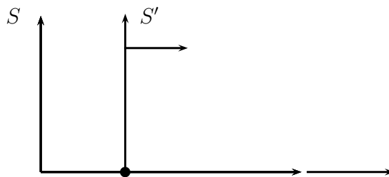
Abbildung 3.9: Punktladung q ruht im Ursprung von S'
