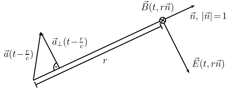
Abbildung 3.52: Strahlungsfeld einer nichtrelativistischen beschleunigten Ladung
