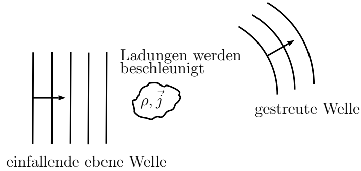
Abbildung 3.57: Schema eines typischen Streuexperimentes
