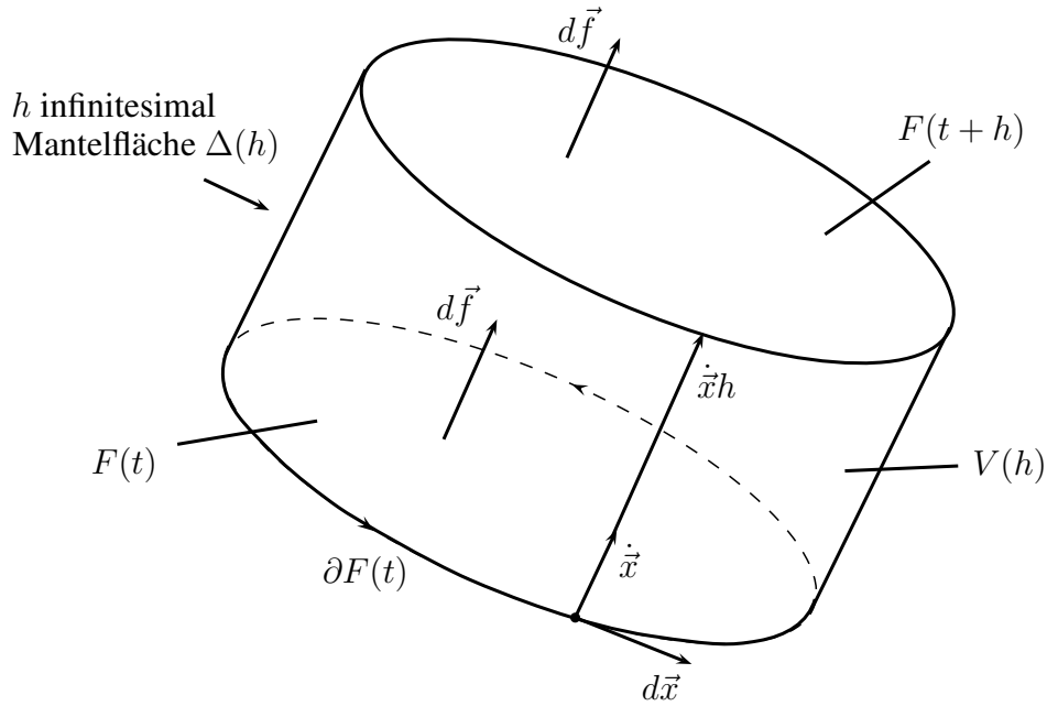
Abbildung 3.36: Bewegung der Integrationsfläche zwischen den Zeitpunkten t und t + h
