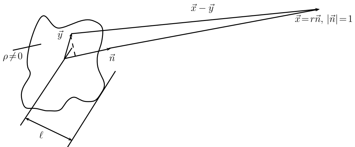
Abbildung 3.14: Elektrisches Feld in großer Entfernung von einer Ladungsverteilung
