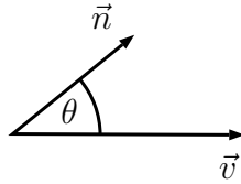
Abbildung 3.55: Ein beschleunigtes ultrarelativistisches Teilchen strahlt hauptsächlich in einen kleinen Winkelbereich um den Geschwindigkeitsvektor
