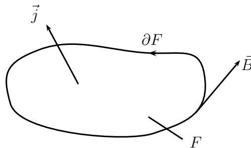
Abbildung 3.19: Illustration von \text{rot } \vec{B} = \frac{4\pi}{c} \vec{j}
