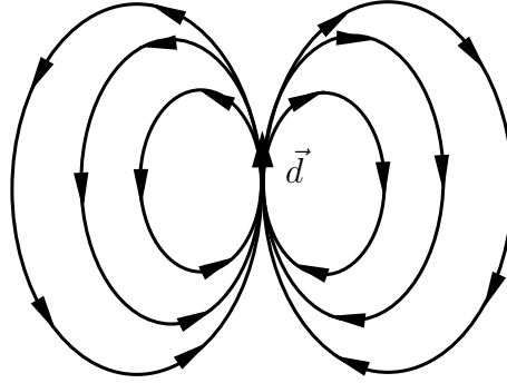
Abbildung 3.16: Elektrisches Feld eines Dipols
