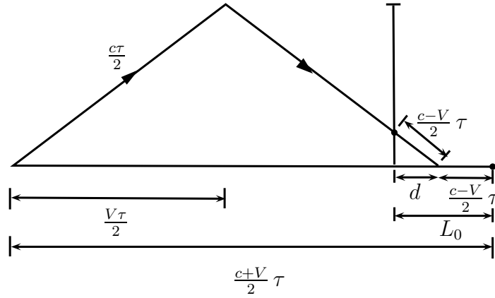
Abbildung 2.7: Bewegte Lichtuhr vom System S aus gesehen. Die Abbildung zeigt die Lichtuhr in jenem Augenblick, in dem das sich horizontal bewegende Photon gerade am rechten Spiegel reflektiert wird
