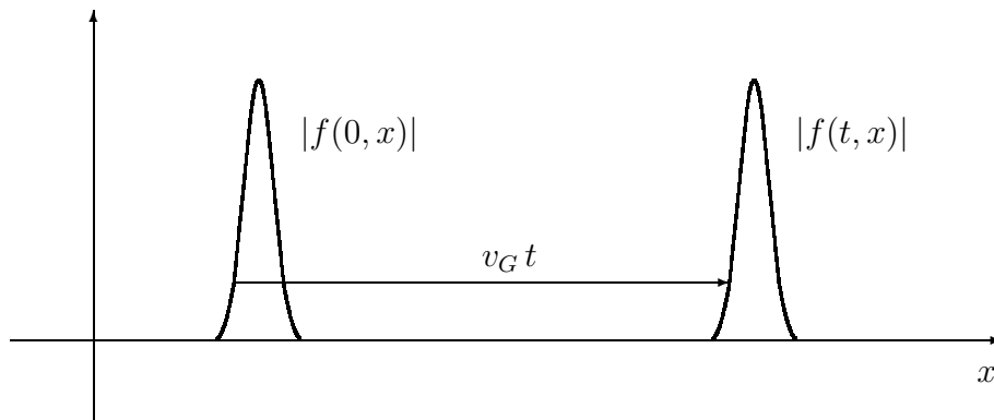
Abbildung 4.35: Räumliche Verschiebung des Wellenpakets mit Gruppengeschwindigkeit v_G
