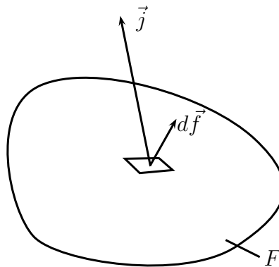
Abbildung 3.3: Stromdichte
