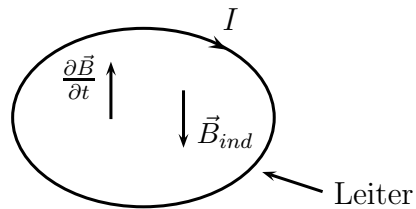
Abbildung 3.40: Lenzsche Regel
