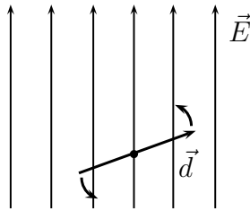
Abbildung 3.18: Dipol in einem homogenen elektrischen Feld
