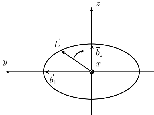
Abbildung 3.45: Elliptisch polarisierte Welle mit Ausbreitung in Richtung der positiven x -Achse (in die Zeichenebene hinein); der Vektor \vec{b}_2 zeigt in Richtung der positiven z -Achse → \vec{E} -Vektor dreht sich im Uhrzeigersinn
