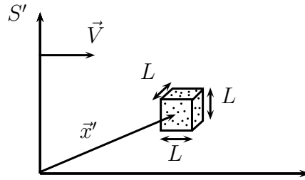
Abbildung 3.7: In S' ruhende Ladung Q in Würfel mit Kantenlänge L
