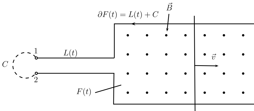
Abbildung 4.27: Konstantes Magnetfeld, bewegter Draht
