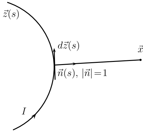
Abbildung 3.24: Stromdurchflossener Draht
