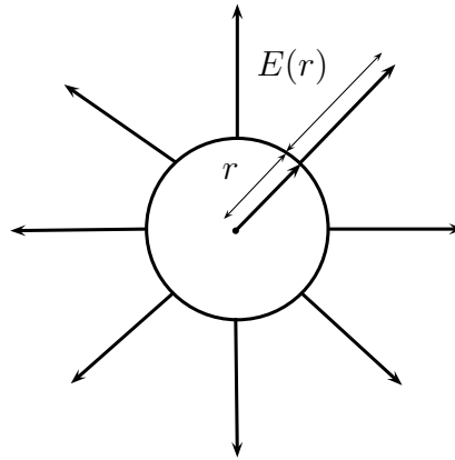
Abbildung 3.8: Elektrisches Feld einer im Ursprung ruhenden Punktladung
