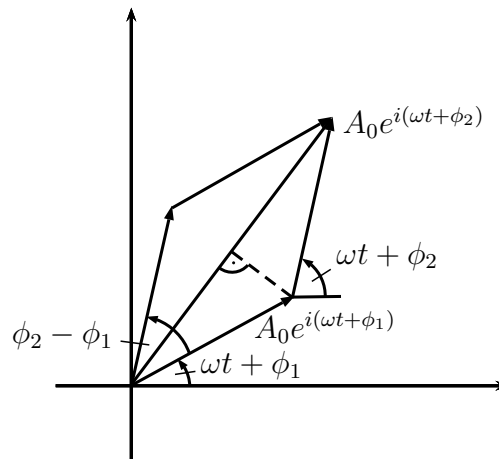
Abbildung 3.59: Ermittlung der resultierenden Amplitude A_R durch Addition komplexer Amplituden
