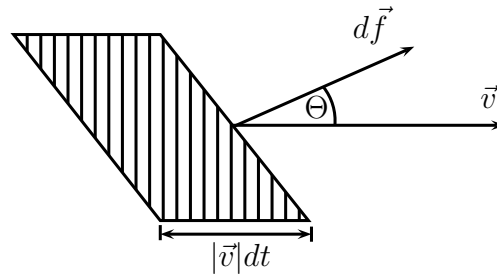
Abbildung 3.4: Geschwindigkeitsfeld
