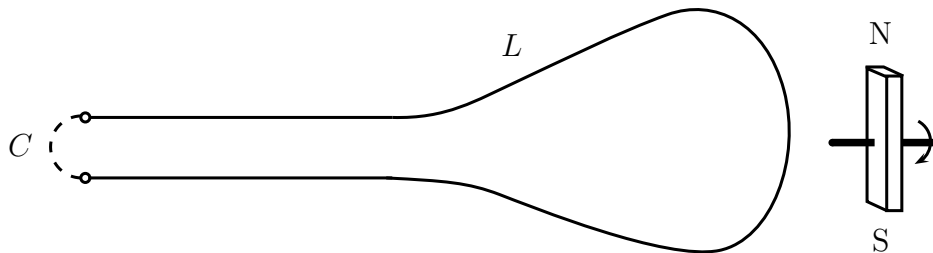
Abbildung 3.34: Ruhende Leiterschleife, zeitlich veränderliches Magnetfeld
