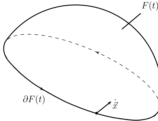
Abbildung 3.35: Zeitlich veränderliche Fläche F(t)
