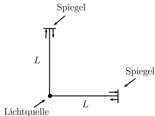
Abbildung 2.6: Modifizierte, in S' ruhende Lichtuhr
