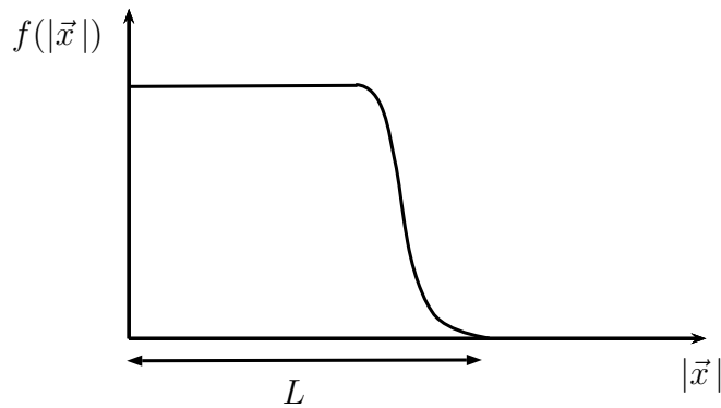
Abbildung 4.1: Mittelungsfunktion
