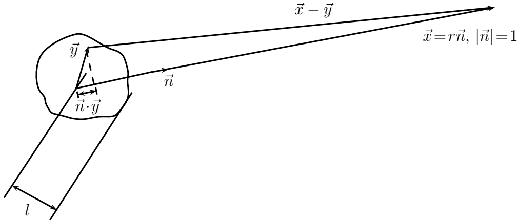
Abbildung 3.50: Zur Berechnung des Strahlungsfeldes in der Fernzone
