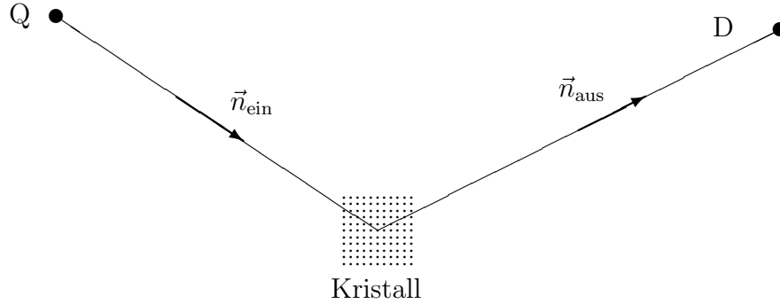
Abbildung 3.64: Streuung von Röntgenstrahlen an einem Kristall
