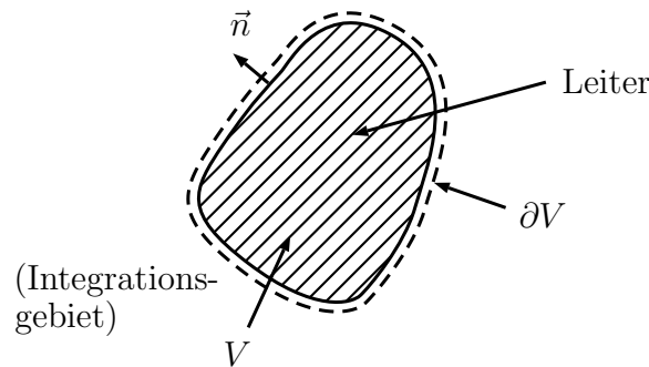
Abbildung 4.11: Kraft auf einen Leiter
