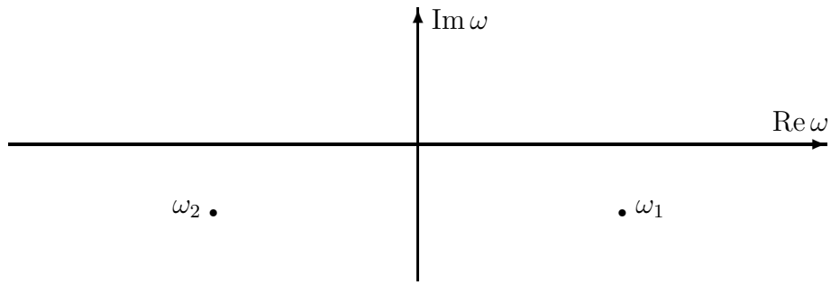
Abbildung 4.30: Pole von \tilde{\varepsilon}(\omega) im Oszillatormodell in der komplexen \omega -Ebene
