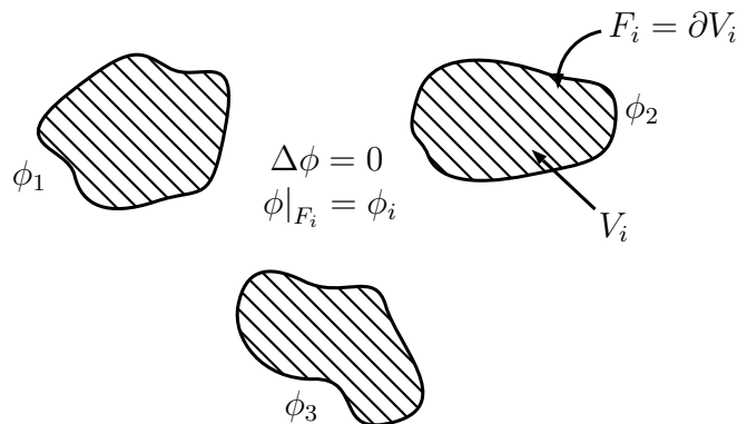
Abbildung 4.4: Randwertproblem in der Elektrostatik von Leitern. Der Raum zwischen den Leitern ist ladungsfrei
