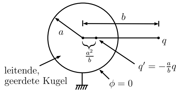
Abbildung 4.15: Geerdete leitende Kugel
