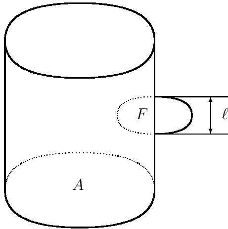
Abbildung 4.23: Strom I_F durch die Fläche F
