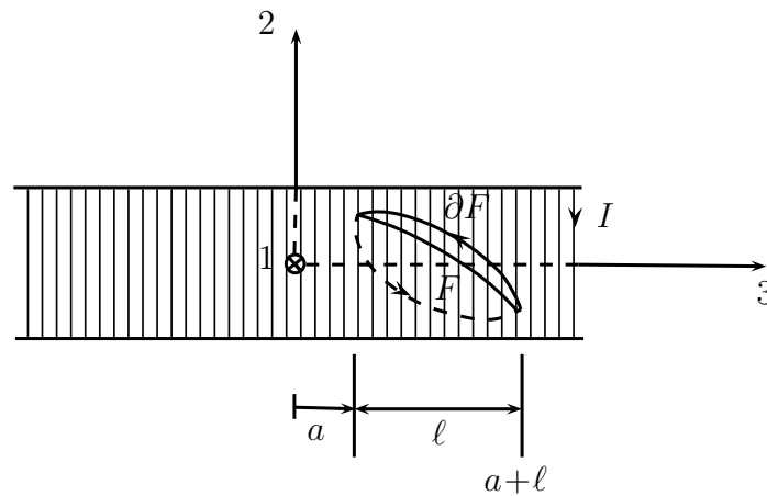
Abbildung 3.27: Fläche F , welche die Oberfläche der Spule durchschneidet
