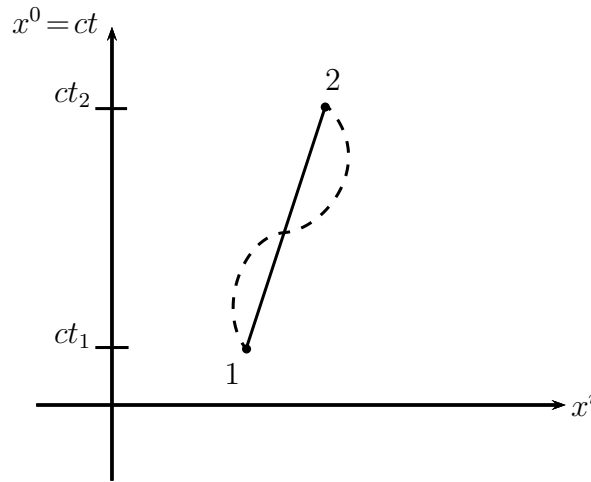
Abbildung 2.11: Variationsproblem zur Ermittlung der Weltlinie eines freien Teilchens in einem Inertialsystem
