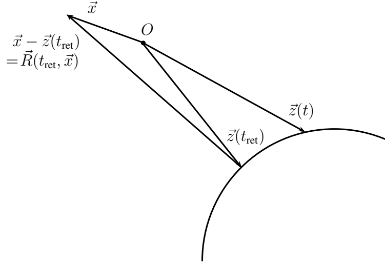
Abbildung 3.53: Das geladene Teilchen bewegt sich auf der Trajektorie t \rightarrow \vec{z}(t) . Das zum Zeitpunkt t am Ort \vec{x} gemessene elektromagnetische Feld wird durch den Beschleunigungs- und Geschwindigkeitsvektor der Ladung zum retardierten Zeitpunkt t_{\text{ret}} bestimmt
