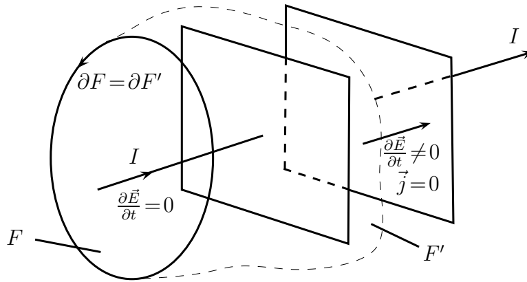
Abbildung 3.39: Maxwell'scher Verschiebungsstrom
