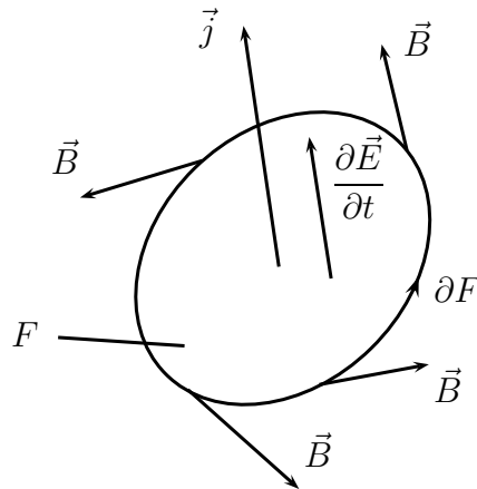
Abbildung 3.38: Erzeugung eines Magnetfeldes durch einen Strom oder ein zeitlich veränderliches elektrisches Feld
