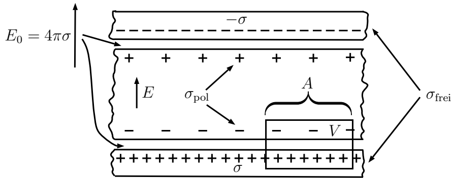
Abbildung 4.17: Plattenkondensator mit Dielektrikum
