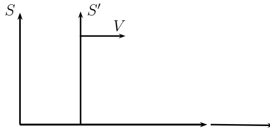
Abbildung 2.8: System S' bewegt sich relativ zu S mit der Geschwindigkeit V
