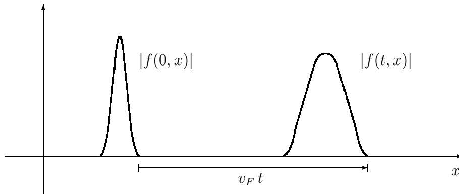
Abbildung 4.36: Frontgeschwindigkeit v_F
