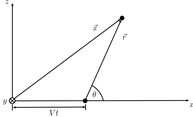
Abbildung 3.10: Radiusvektor \vec{r}
