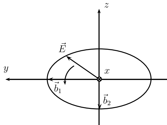
Abbildung 3.46: Elliptisch polarisierte Welle mit Ausbreitung in Richtung der positiven x -Achse (in die Zeichenebene hinein); der Vektor \vec{b}_2 zeigt in Richtung der negativen z -Achse → \vec{E} -Vektor dreht sich gegen den Uhrzeigersinn
