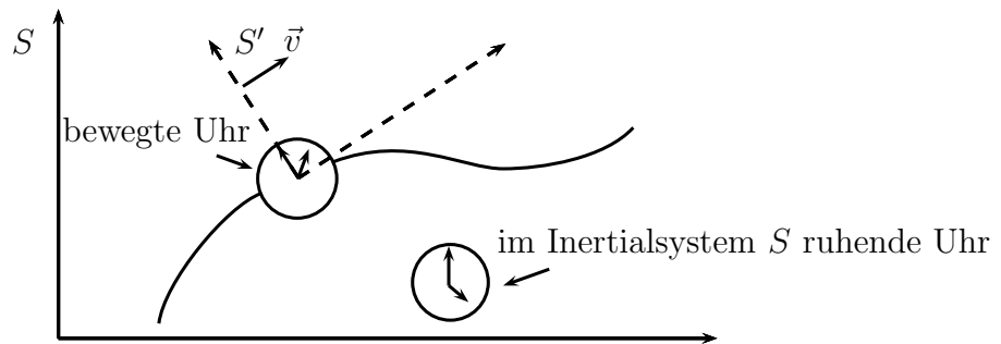
Abbildung 2.10: Beliebige bewegte Uhr
