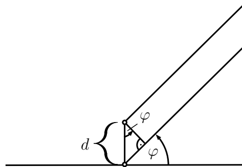
Abbildung 3.60: Zwei Dipoloszillatoren im Abstand d
