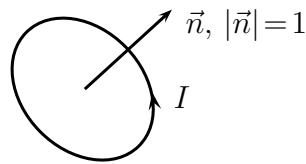
Abbildung 3.30: Rechte-Hand-Regel
