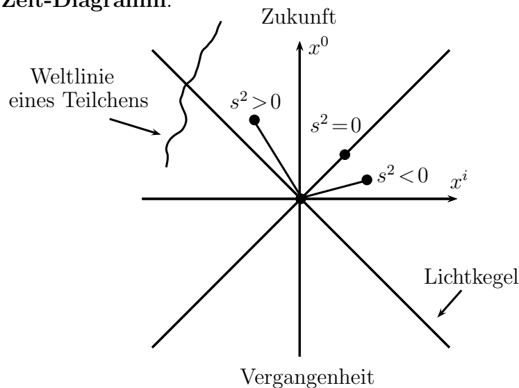
Abbildung 2.9: Raum-Zeit-Diagramm
