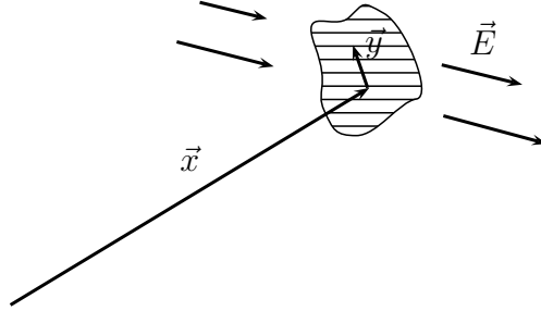
Abbildung 3.17: Ladungsverteilung in einem äußeren elektrischen Feld \vec{E}
