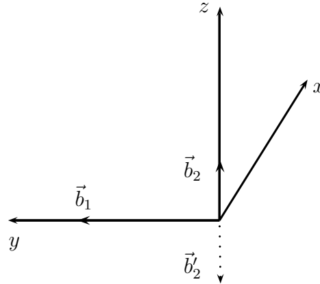
Abbildung 3.44: Monochromatische ebene Welle in Richtung der positiven x -Achse; Wahl der y -Achse in Richtung von \vec{b}_1 ; der auf \vec{b}_1 normal stehende Vektor \vec{b}_2 kann entweder in Richtung der positiven oder in Richtung der negativen z -Achse weisen
