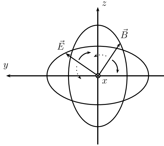
Abbildung 3.47: Elektrisches und magnetisches Feld einer elliptisch polarisierten Welle
