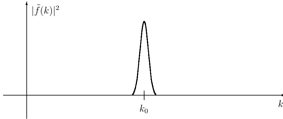
Abbildung 4.34: Spektrum eines fast monochromatischen Wellenpakets
