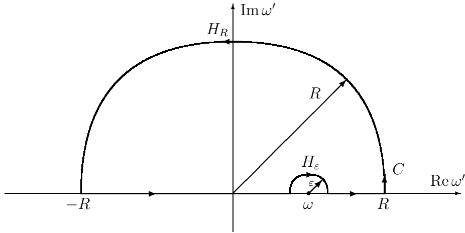
Abbildung 4.31: Wegintegral in der komplexen Ebene
