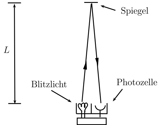
Abbildung 2.3: Lichtuhr
