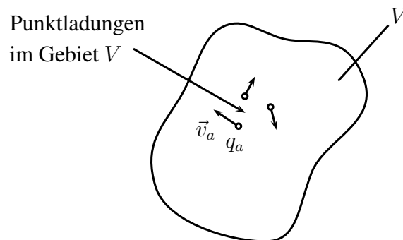
Abbildung 3.41: Punktladungen und elektromagnetisches Feld im Gebiet V
