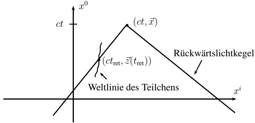
Abbildung 3.54: Die Weltlinie des Teilchens schneidet den Rückwärtslichtkegel nur in einem einzigen Punkt
