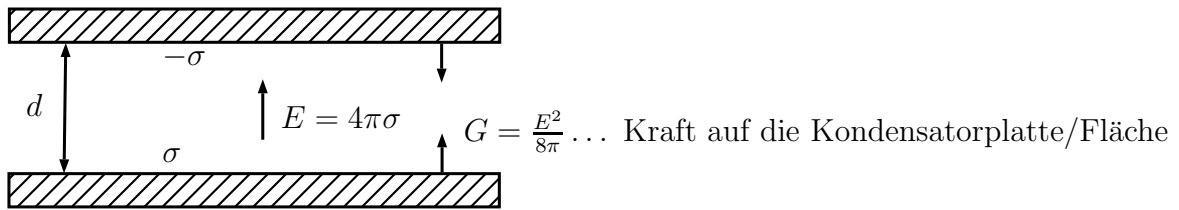
Abbildung 4.12: Flächenkraftdichte auf eine Kondensatorplatte
