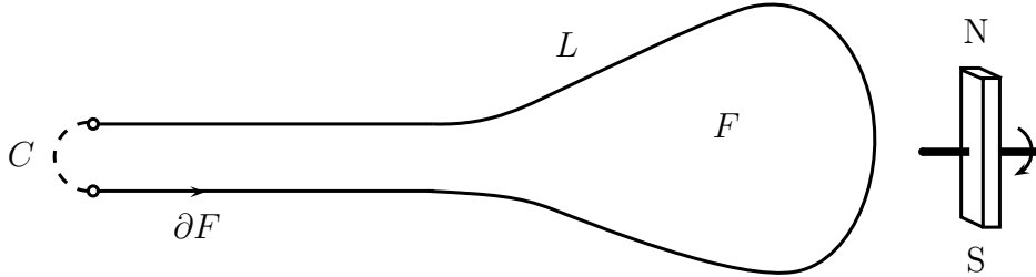
Abbildung 4.26: Induktionsgesetz für ruhende Leiterschleife mit \partial \vec{B} / \partial t \neq 0
