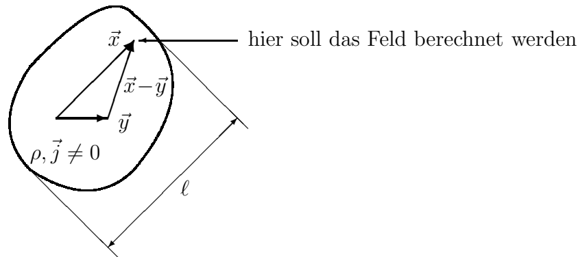
Abbildung 4.24: Berechnung des Feldes in der Nahzone
