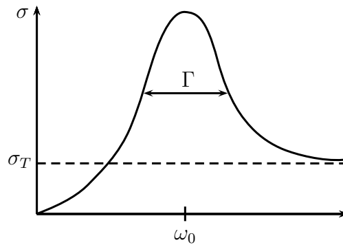
Abbildung 3.58: Streuquerschnitt als Funktion der Kreisfrequenz der einfallenden Welle
