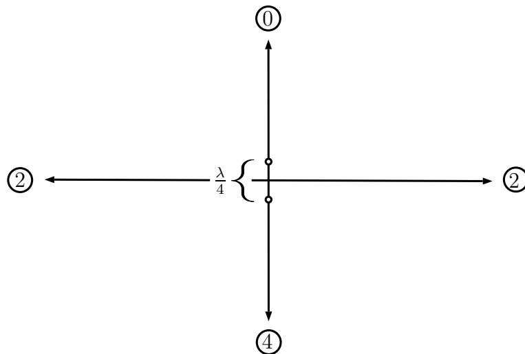
Abbildung 3.63: \phi_2 - \phi_1 = \frac{\pi(\sin \varphi + 1)}{2} , I_2/I_1 = 4 \cos^2 \frac{\pi(\sin \varphi + 1)}{4} (sendet bevorzugt in nur eine Richtung)
