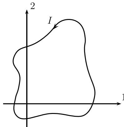
Abbildung 3.26: Spule mit beliebigem Querschnitt
