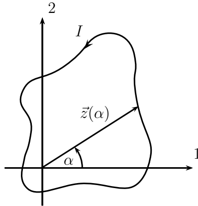
Abbildung 3.29: Magnetisches Dipolmoment einer ebenen Leiterschleife
