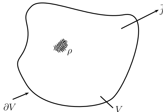
Abbildung 3.5: Interpretation der Kontinuitätsgleichung
