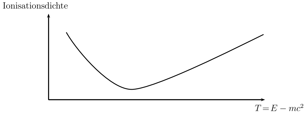
Abbildung 3.13: Ionisationsdichte
