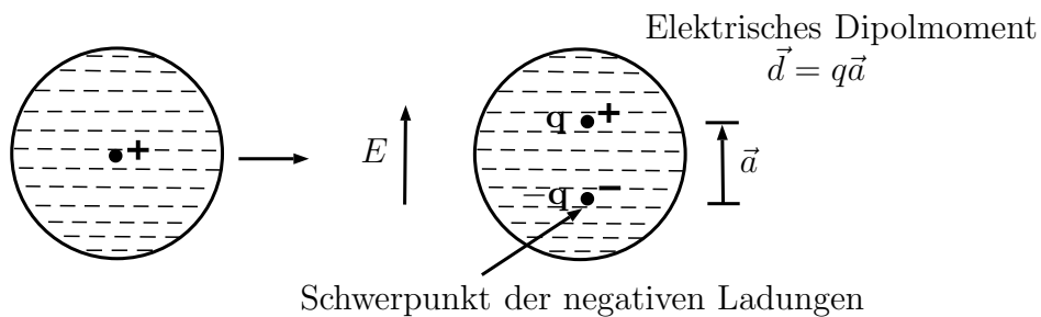
Abbildung 4.18: Neutrales Atom vor und nach dem Anlegen eines äußeren elektrischen Feldes
