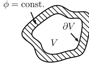
Abbildung 4.5: Faradayscher Käfig
