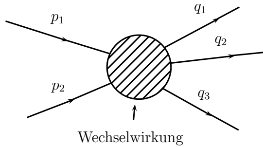
Abbildung 2.12: Schematische Darstellung eines Prozesses in der Teilchenphysik
