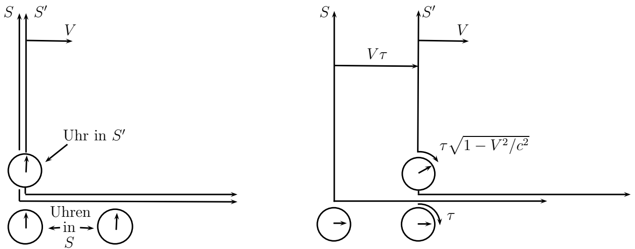
Abbildung 2.2: Zeitdilatation
