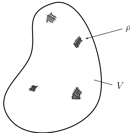
Abbildung 3.2: Ladungsdichte
