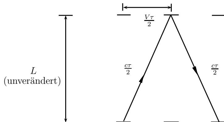
Abbildung 2.4: Bewegte Lichtuhr
