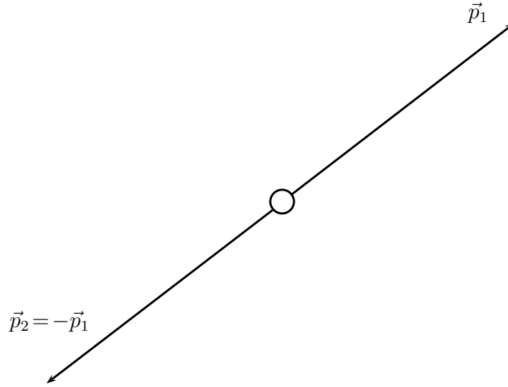
Abbildung 2.14: Impulserhaltung
