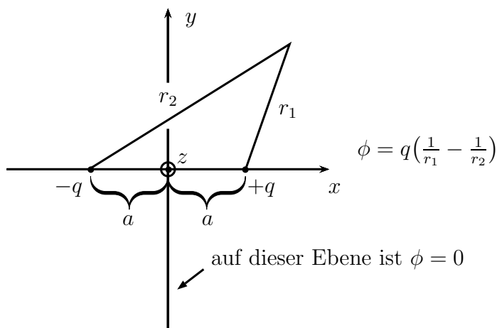
Abbildung 4.13: Potential zweier entgegengesetzt gleich großer Ladungen
