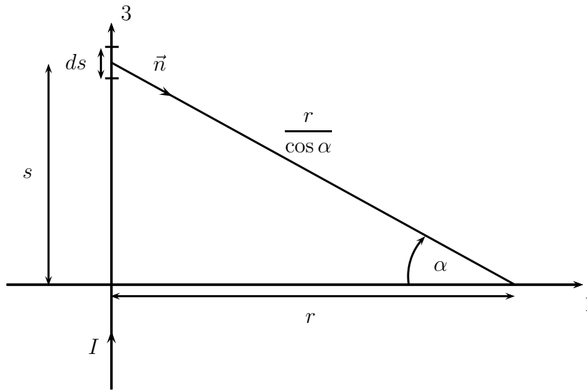
Abbildung 3.25: Berechnung des Magnetfelds mit Hilfe der Formel von Biot-Savart
