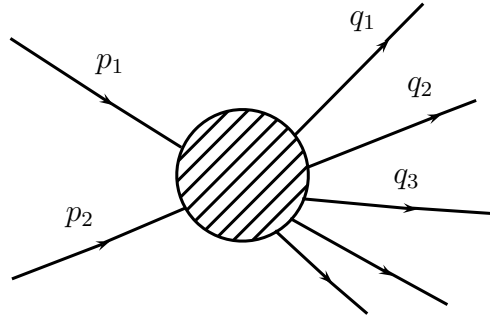
Abbildung 2.15: Erzeugung neuer Teilchen in einem Kollisionsexperiment
