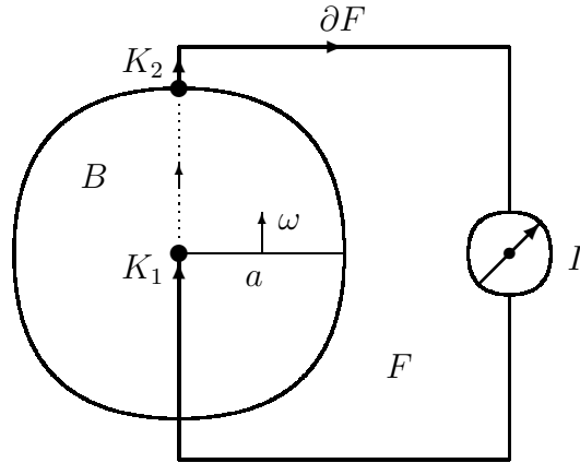
Abbildung 4.29: Metallscheibe mit Radius a rotiert mit Winkelgeschwindigkeit \omega ; normal darauf zeitlich konstantes Magnetfeld B ; Schleifkontakte K_1, K_2
