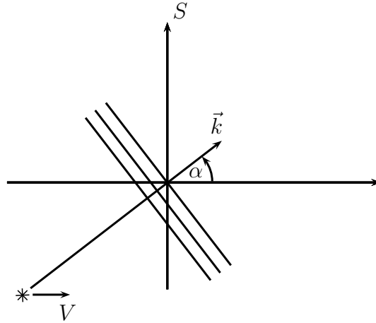
Abbildung 3.48: Ein Stern bewegt sich relativ zu einem Beobachter. \vec{k} ist der Wellenzahlvektor des vom Stern ausgesandten Lichts im System des Beobachters
