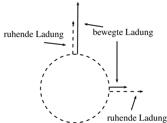
Abbildung 3.11: Elektrisches Feld einer ruhenden und einer bewegten Punktladung
