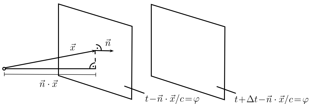
Abbildung 3.42: Flächen konstanter Phase bei einer ebenen Welle
