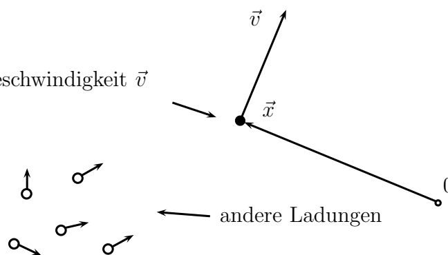
Abbildung 3.1: Probeladung in einem äußeren elektromagnetischen Feld
