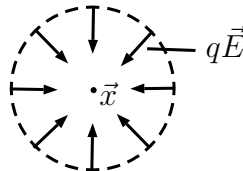
Abbildung 4.6: Kraft auf eine Probeladung bei stabilem Gleichgewicht
