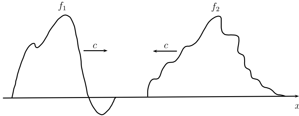
Abbildung 3.43: Allgemeine Lösung der Wellengleichung in einer Raumdimension
