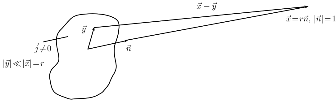
Abbildung 3.28: Multipolentwicklung eines von der Stromverteilung \vec{j} erzeugten Magnetfeldes
