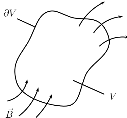
Abbildung 3.20: Illustration von \operatorname{div} \vec{B} = 0
