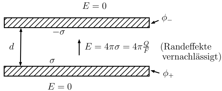
Abbildung 4.7: Plattenkondensator
