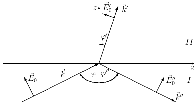
Abbildung 4.37: Reflexion und Brechung an der Grenze zweier Medien
