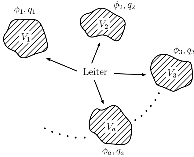
Abbildung 4.10: Zur Berechnung der Feldenergie
