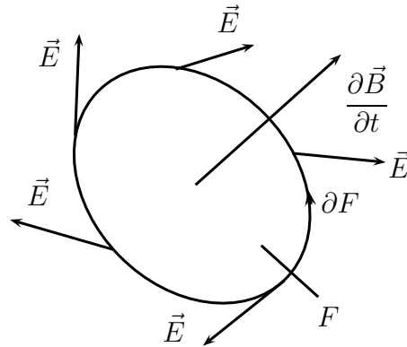
Abbildung 3.33: Induktionsgesetz für eine zeitlich konstante Fläche F
